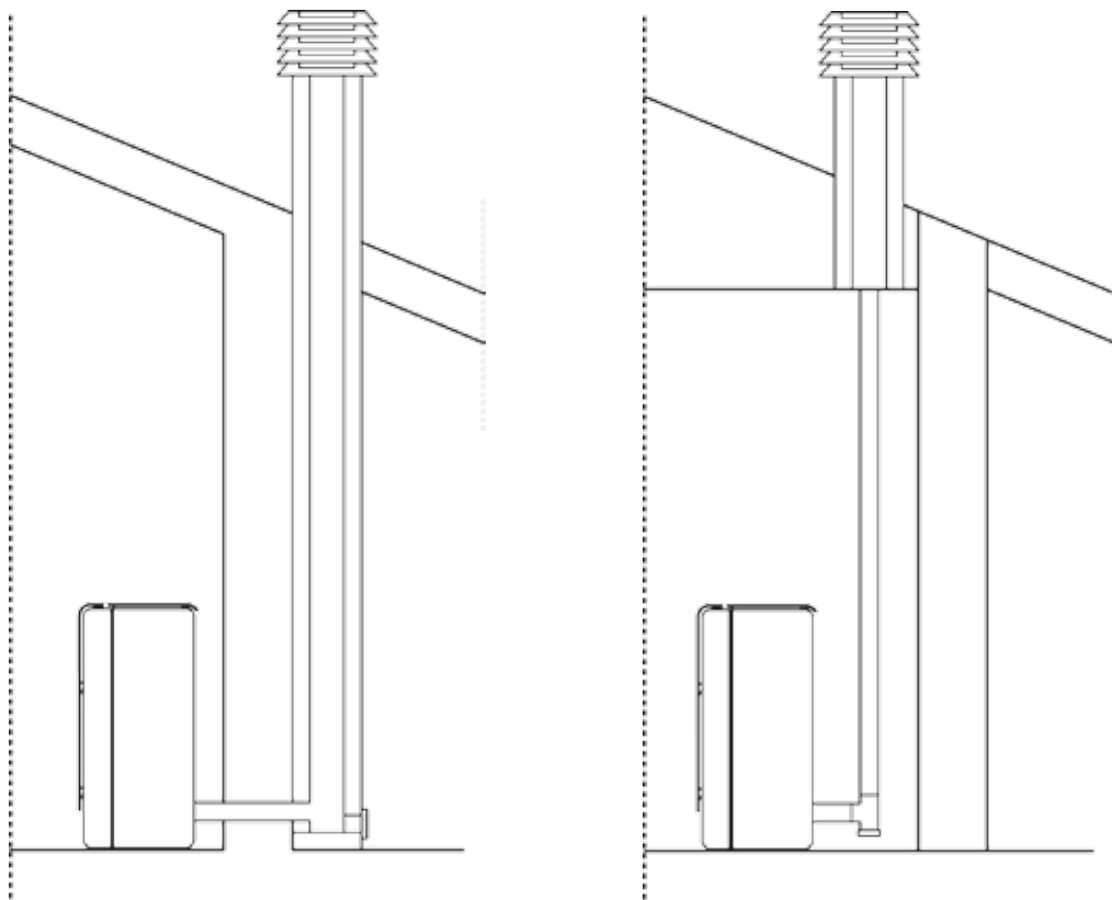
FIGURA - Scarico mediante camino tradizionale
