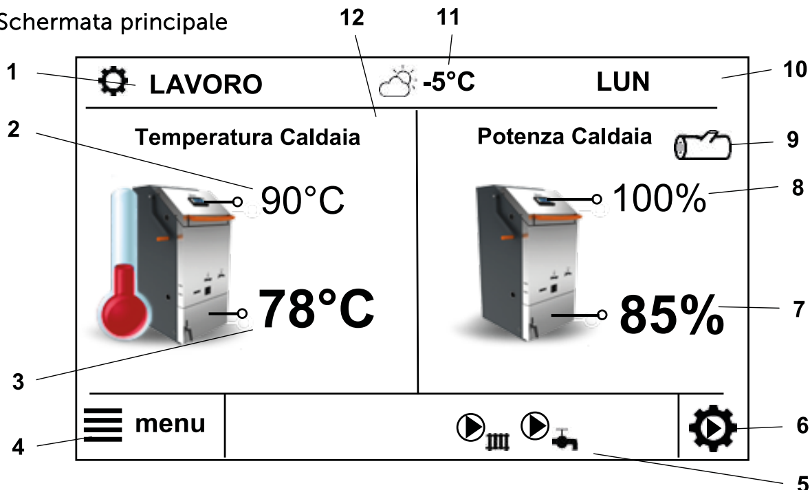
Figura 1. Schermata principale del regolatore
