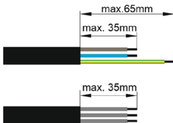
Figura 10. Lunghezza di spelatura del cavo
