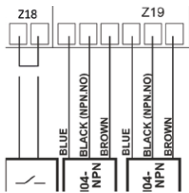
Figura 15. Schema elettrico di collegamento dei sensori induttivi
