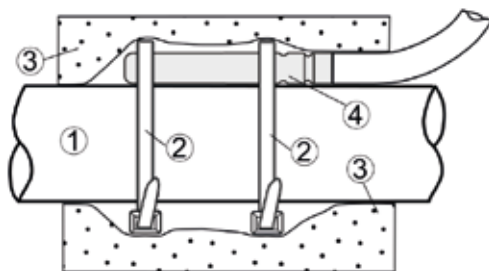
Figura 16. Installazione della sonda di temperatura sul tubo,
