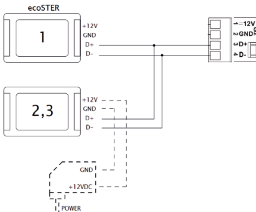
Figura 25. Collegamento combinato del pannello ambiente ecoSTER
