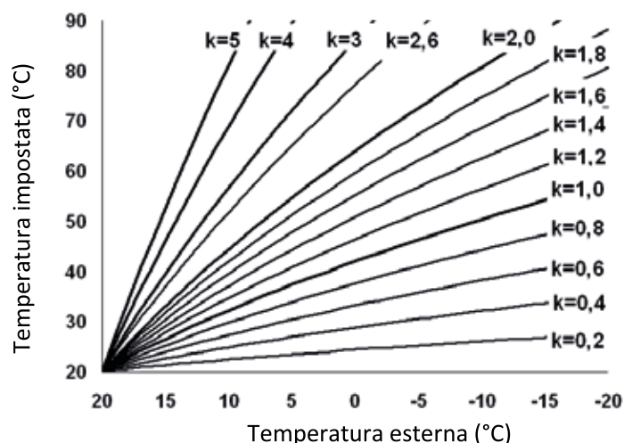
Figura 6. Curve climatiche
