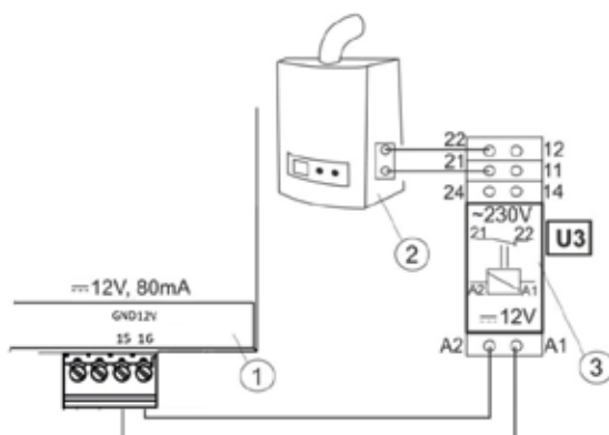
Figura 26. Collegamento elettrico della caldaia di riserva:
