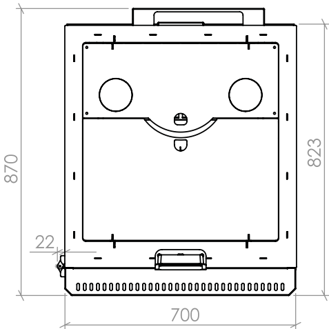
VISTA SUPERIORE
